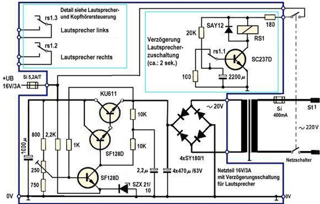
Schaltbild: Netzteil 16V/3A mit Lautsprechersteuerung
