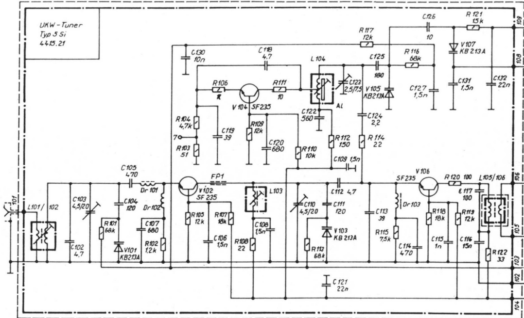
Schaltplan: UKW-Tuner-Typ5/Si
