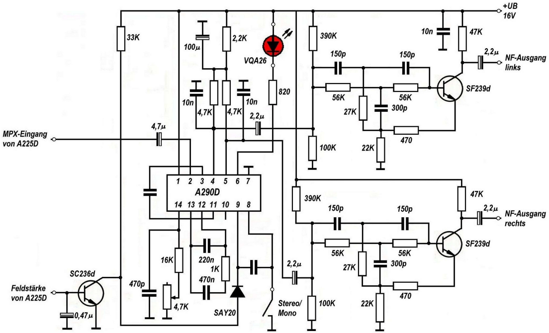
Schaltbild Stereodekoder AM/FM - Empfänger
