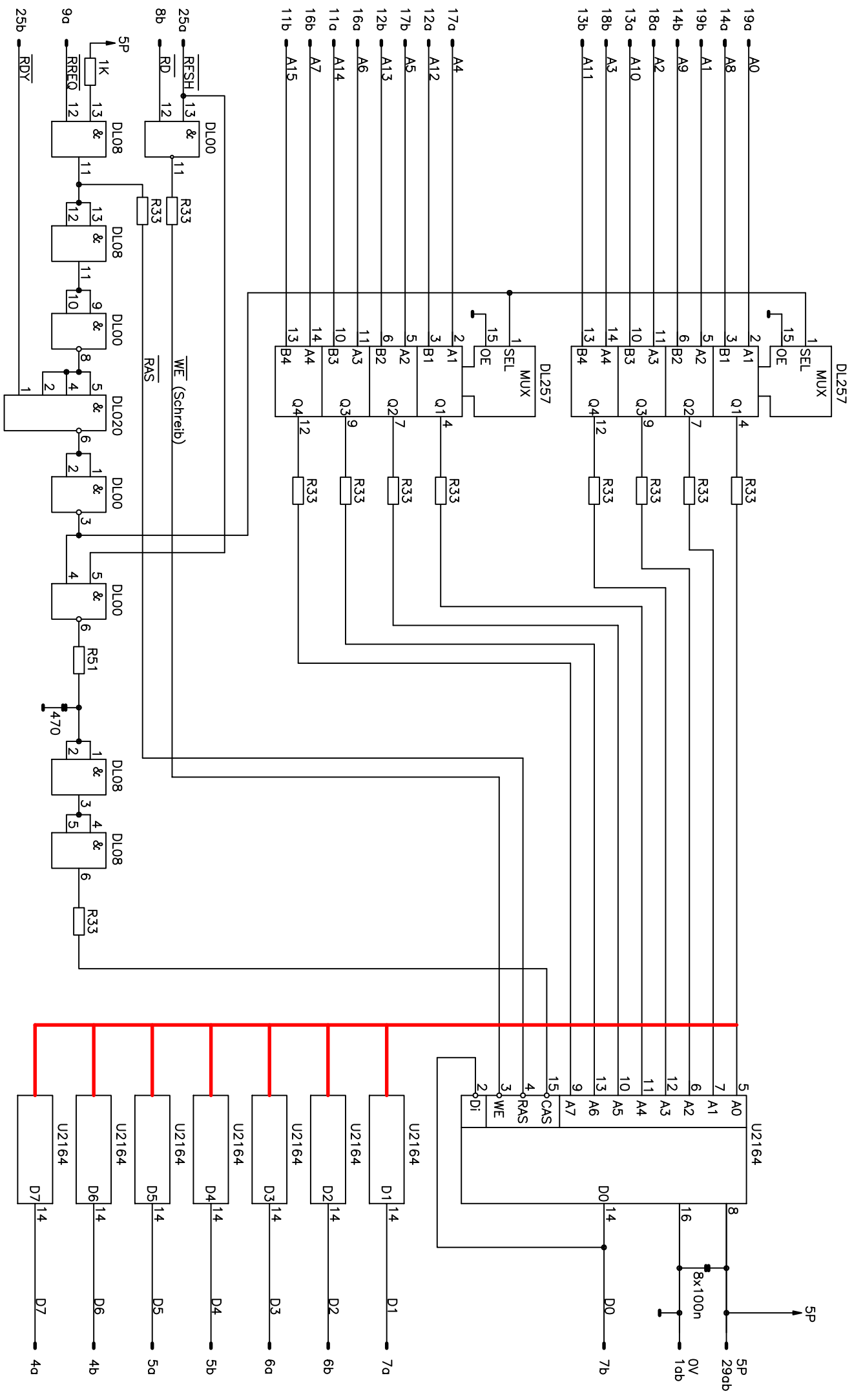
AC1 – 64K dynamischer RAM Kontaktbezeichnung nach Jahn EGS-AC1/V3
