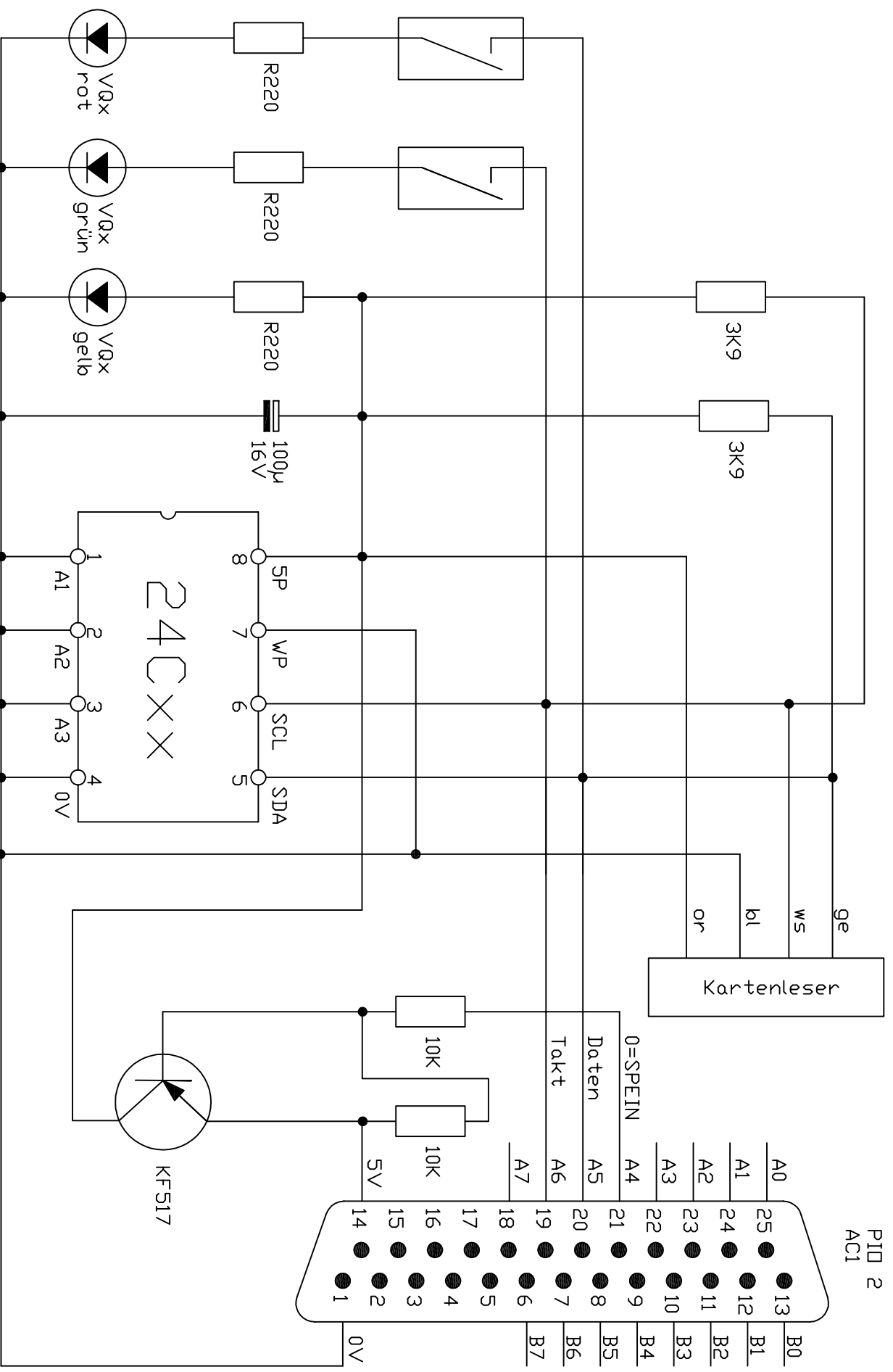
Versuchsschaltung Lesen 24C02-24C256
